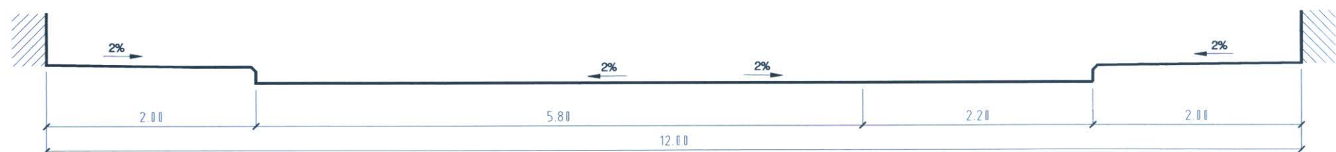
VIAL TIPO 2 - C/ PROLONGACION LA CLOSA - C/ EN PROYECTO 1
